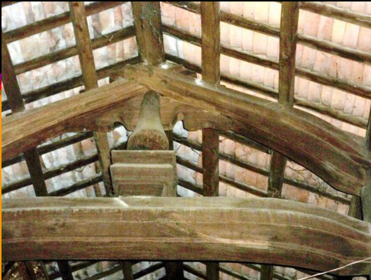
Bộ khung tại đình Bình Hòa – Giồng trôm, Bến Tre
